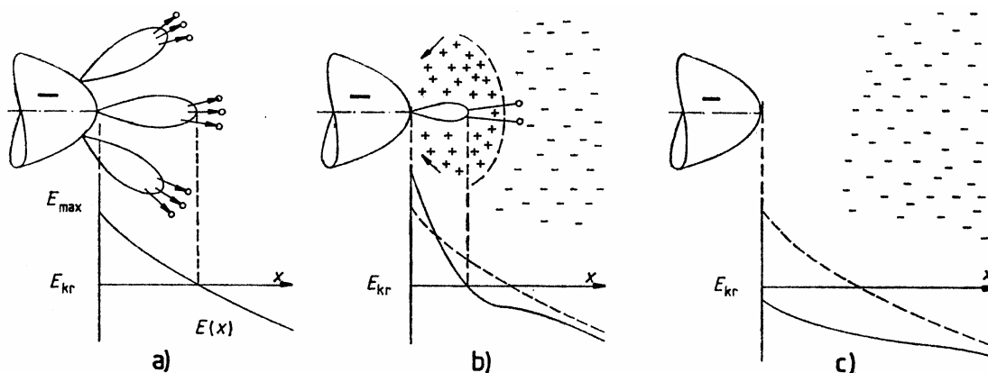
Koronakisülés negatív csúcson: a negatív elektród előtt egy nagy negatív töltésfelhő alakul ki. Sok idő alatt a másik elektród kiszippantja ezeket.
