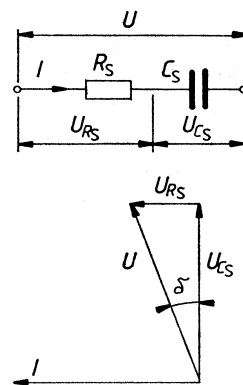
Soros helyettesítő kapcsolás
