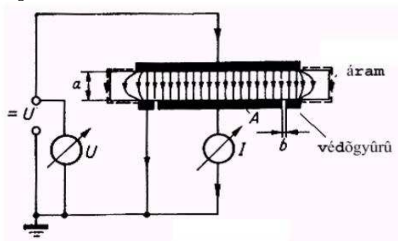
Fajlagos térfogati ellenállás mérésére szolgáló elrendezés
