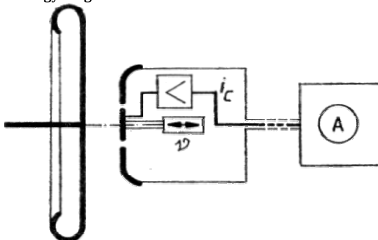
Rezgőkondenzátoros voltmérő elvi felépítése
