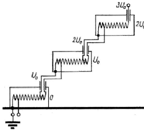
Kaszkád transzformátor kapcsolása
