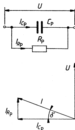
Párhuzamos helyettesítő kapcsolás
