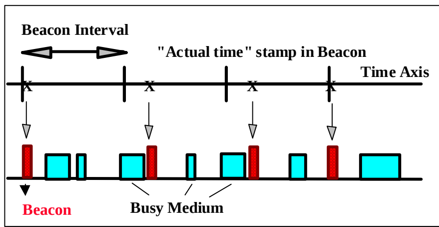
2.20. ábra Beacon jelek átvitelének folyamata
