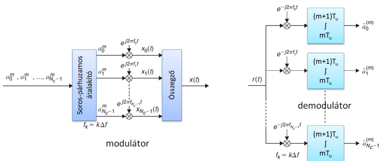
3.3.ábra – OFDM modulátor (bal) és demodulátor (jobb) [2]
