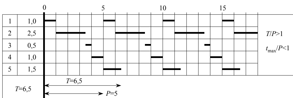
4.3/b. ábra: Kis- és középsorozat-gyártás
