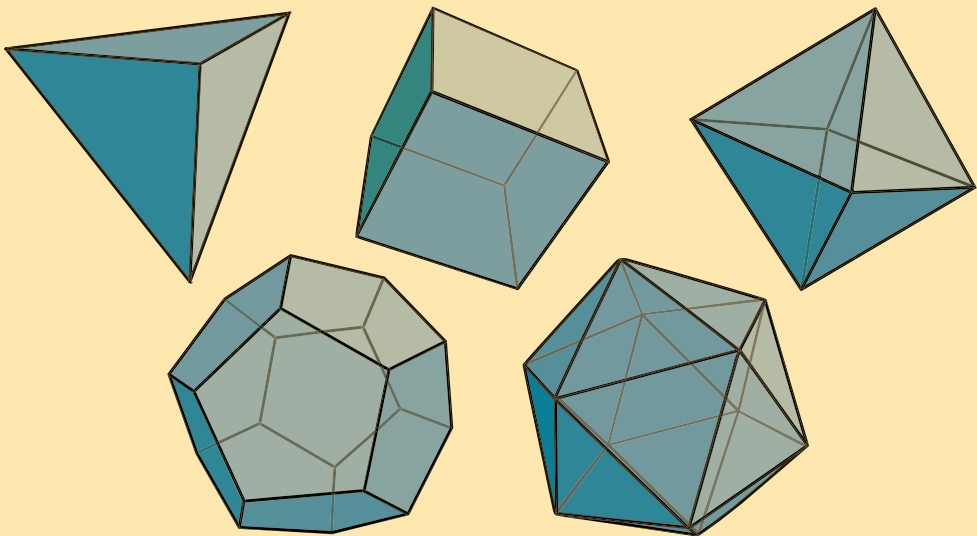
3.9. ábra A szabályos testek
