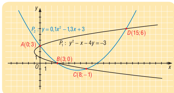
4.12. ábra A példában szereplő parabolák és metszéspontjaik
