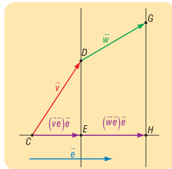
6.4. ábra „ \vec{e}\vec{v} + \vec{e}\vec{w} ”
