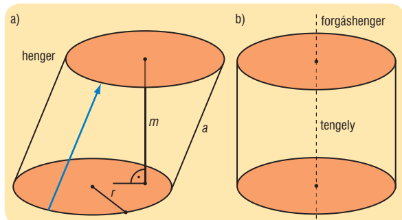
4.4. a) b) ábra Hengerek
