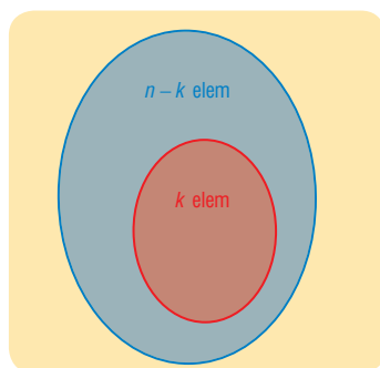
3.3. ábra A k elemű részhalmazok száma
