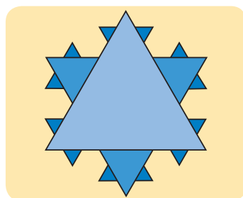
6.8. ábra A Koch-féle hópehely első néhány háromszöge
