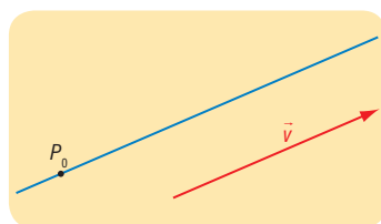
2.4. ábra Egyenes és irányvektora
