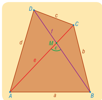
5.8. ábra Konvex négyszög
