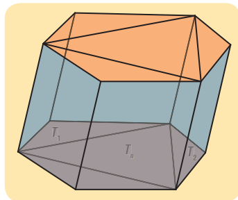
9.6. ábra Hasáb térfogata
