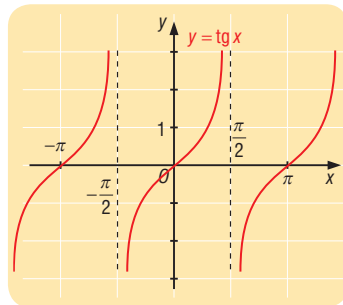
14.4. ábra A tangensfüggvény grafikonja
