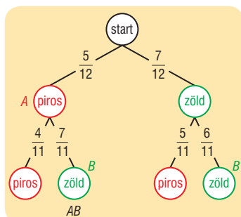
5.2. ábra A 2. b) példa gráfja
