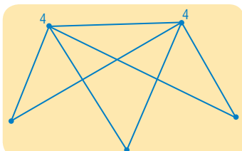
5.5. ábra Minden pont fokszáma legalább 2
