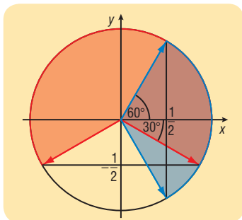
9.9. ábra Az I. feltétel ábrázolása egységkörön
