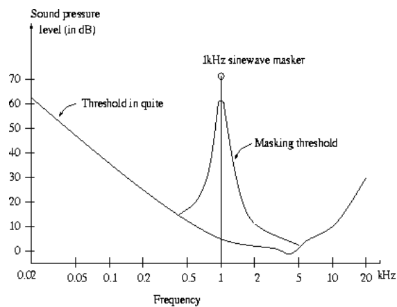
Egy 1 kHz-es szinuszjel maszkoló hatása
