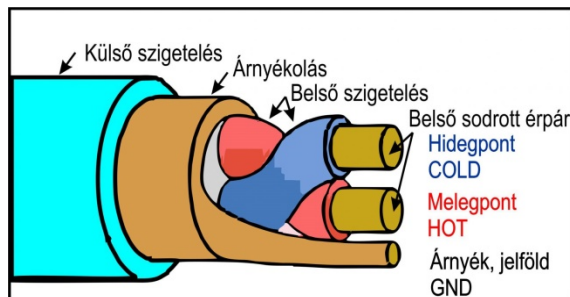
Csavart érpár / szimmetrikus kábel felépítése
