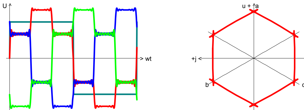
Az egyszerű inverter feszültsége, a számításba vett harmonikusok száma: 15
