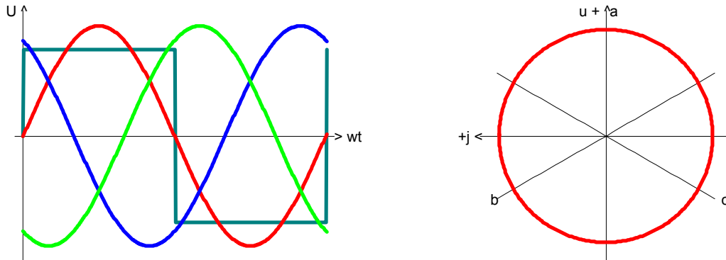
Az egyszerű inverter feszültsége, a számításba vett harmonikusok száma: 1
