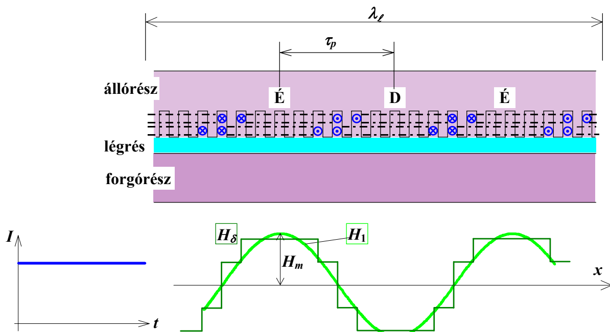
Kétrétegű tekercs lépcsős mágneses tere a kiterített légrésben egyenáramú táplálásnál
