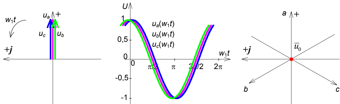
Zérus sorrendű feszültségrendszer fázorábrája időfüggvénye Park-vektora
