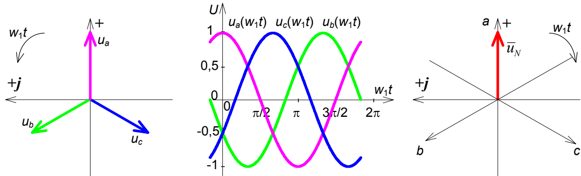
Negatív sorrendű feszültségrendszer fázorábrája időfüggvénye Park-vektora
