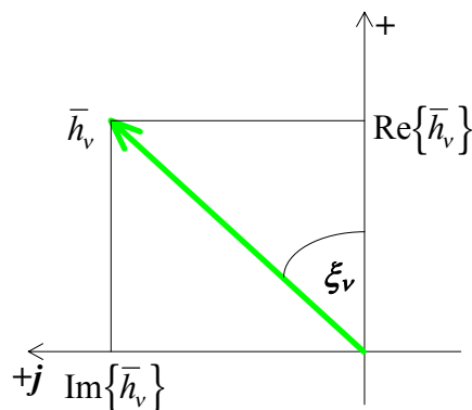
A Park-vektor v. harmonikus összetevője
