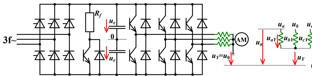
Egyszerű inverterről táplált aszinkron motor áramköri vázlata
