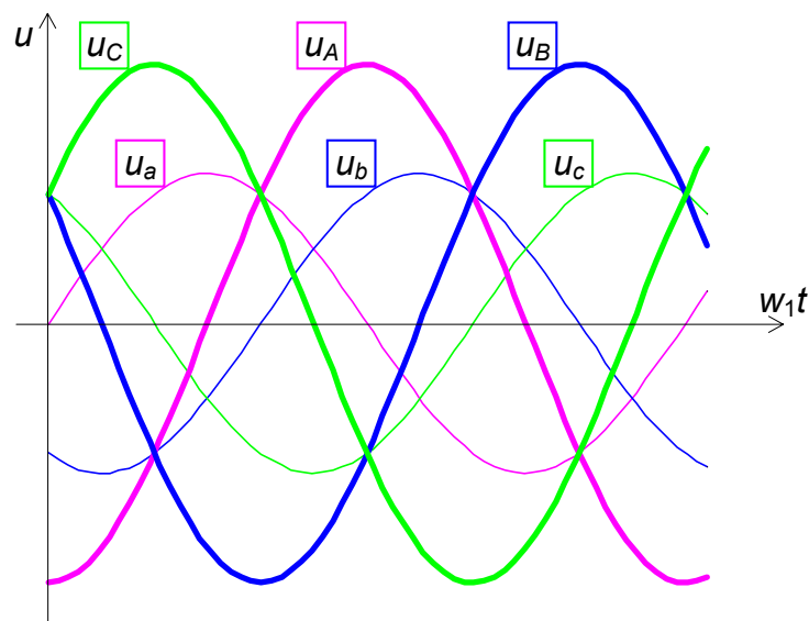
A fázis- és vonali feszültségrendszer időfüggvénye
