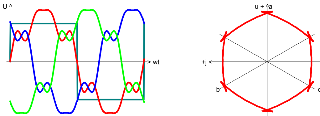
Az egyszerű inverter feszültsége, a számításba vett harmonikusok száma: 3
