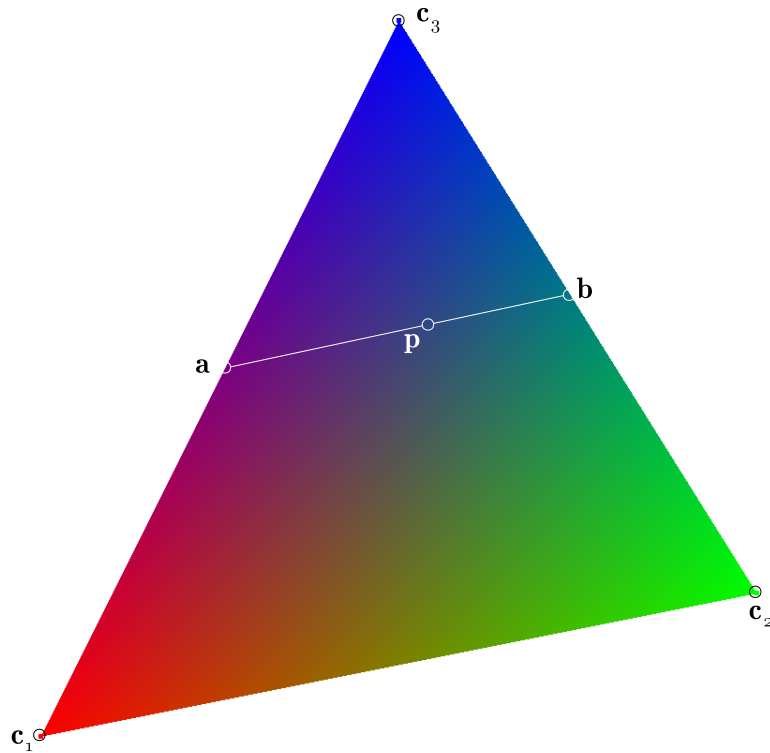
4.3. ábra. Gouroud-féle árnyalás
