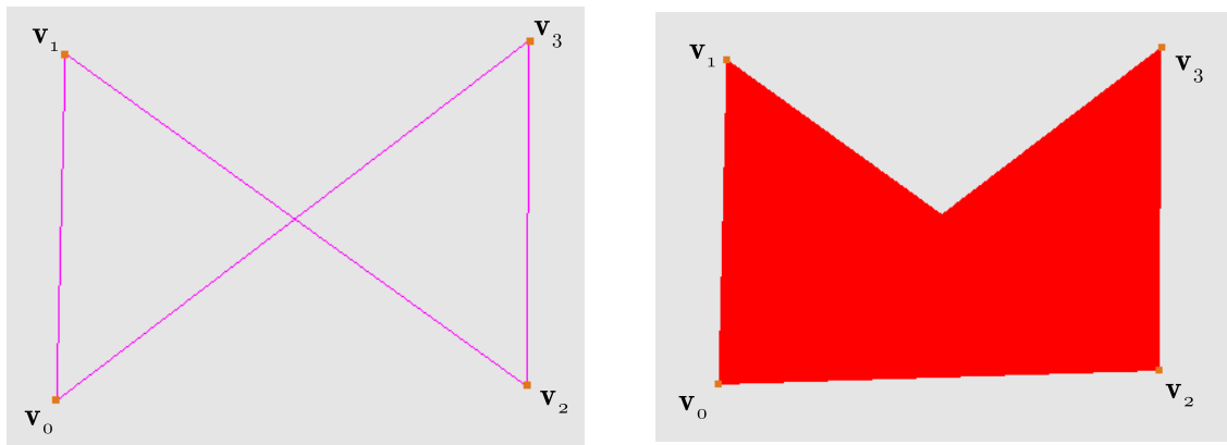
3.4. ábra. Nem komplanáris csúcspontú négyszög vetületei; a bal oldali ábrán az éleivel, a jobb oldalin mindkét oldalát kifestve ábrázolva
