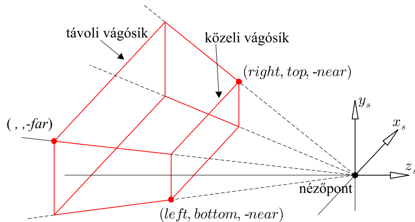
5.2. ábra. A glFrustum ( ) függvény paramétereinek jelentése
