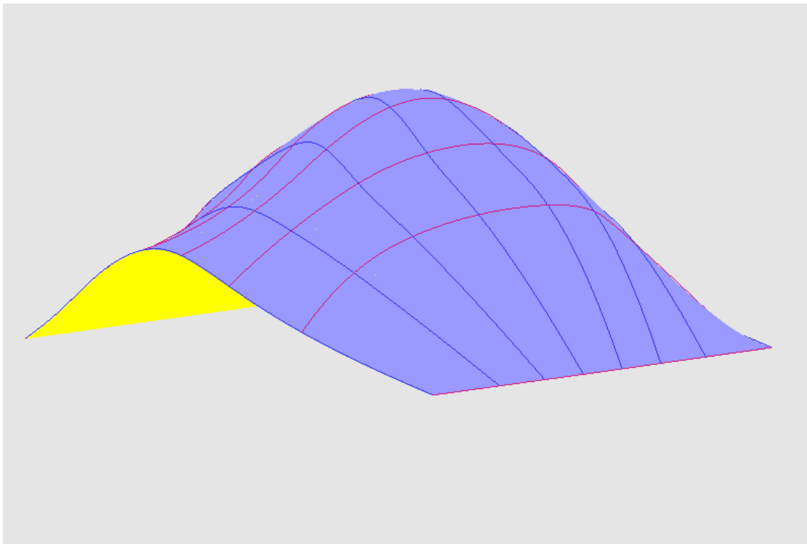
15.6. ábra. A felület és a paramétervonalával ekvidisztáns görbék
