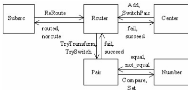
6.13. ábra: Eseményfolyam diagram.
