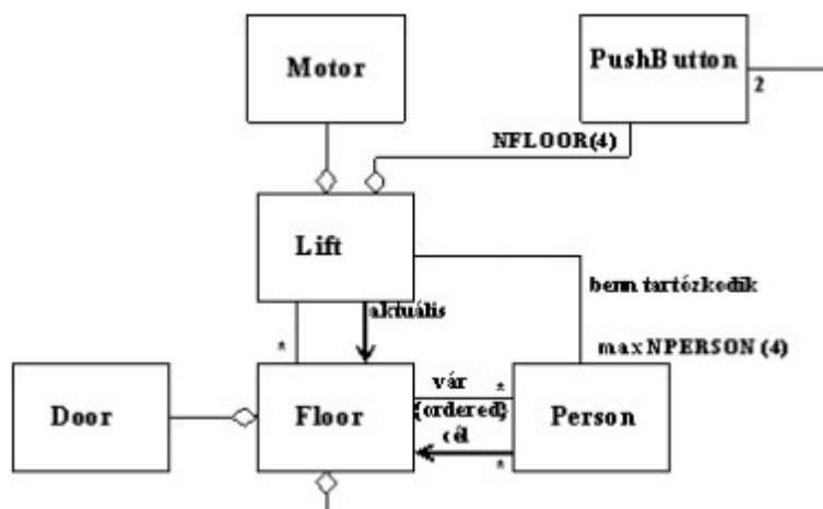
8.9. ábra: A lift feladat osztálydiagramja.
