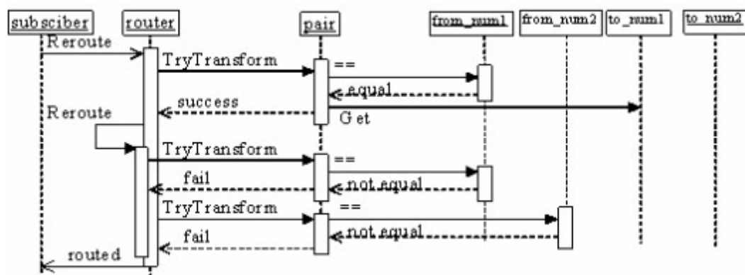
6.5. ábra: Szám átírányítása
