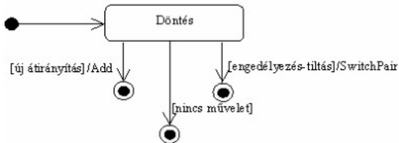
6.15. ábra: A központ módosított állapottér modellje.
