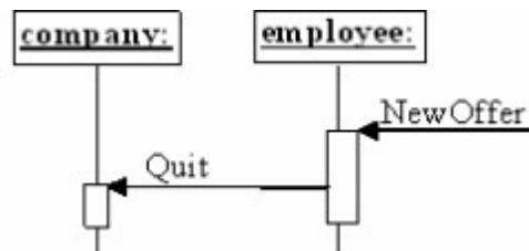
7.5. ábra: Üzenet előzmény nélkül.
