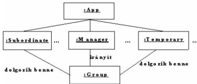
8.3. ábra: Az irodai hierarchia program objektumdiagramja
