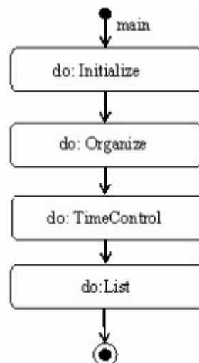
8.6. ábra: Az applikációs program állapotgépe.
