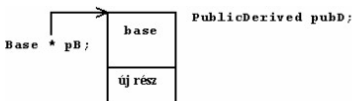
6.24. ábra: Szűkítő típuskonverzió.
