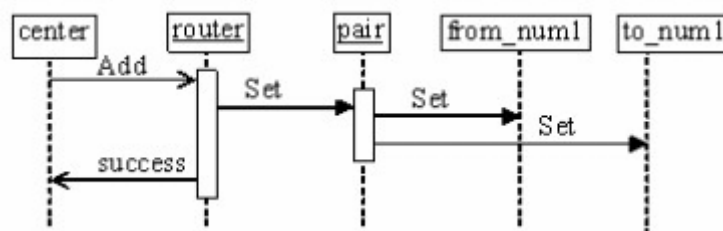
6.7. ábra: Új számpár felvétele
