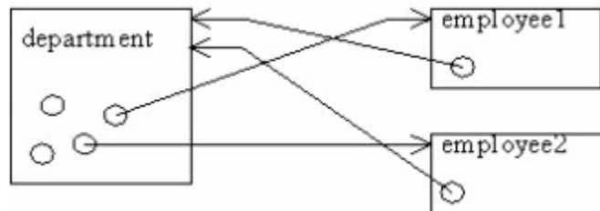
7.7. ábra: Redundáns asszociációk.
