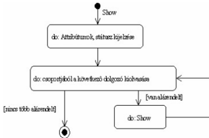
8.5. ábra: A menedzser állapottér modellje
