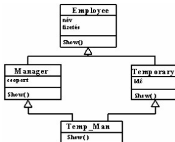
6.21. ábra: Többszörös öröklés.
