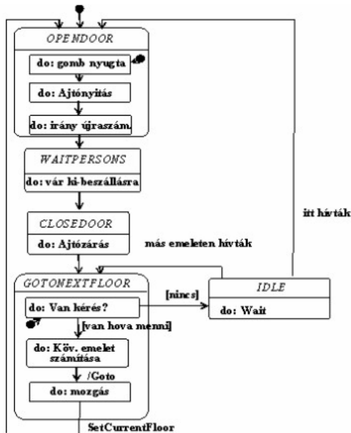
8.13. ábra: A lift állapottér modellje.
