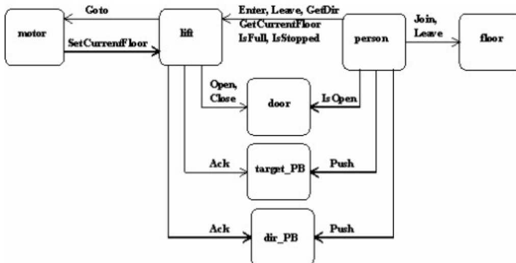
8.15. ábra: Láthatósági viszonyok.
