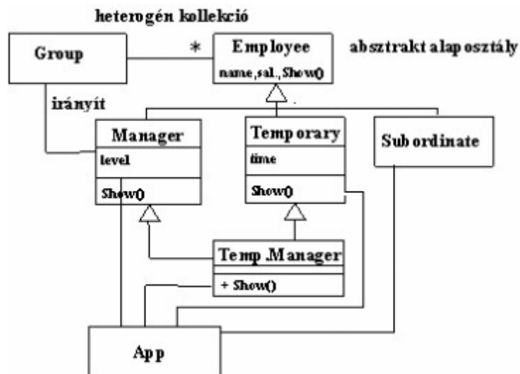
8.2. ábra: Az irodai hierarchia program osztálydiagramja
