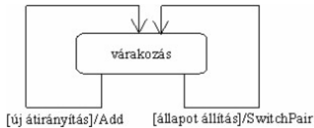
6.11. ábra: A router objektum dinamikus modellje új átirányítás, illetve állapot állítás esetén.
