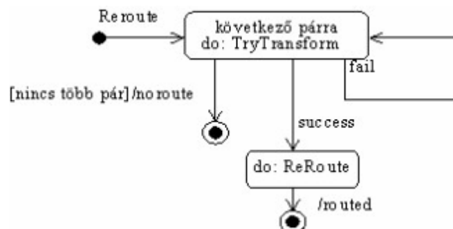
6.9. ábra: A router objektum dinamikus modellje. A Reroute üzenet hatása.
