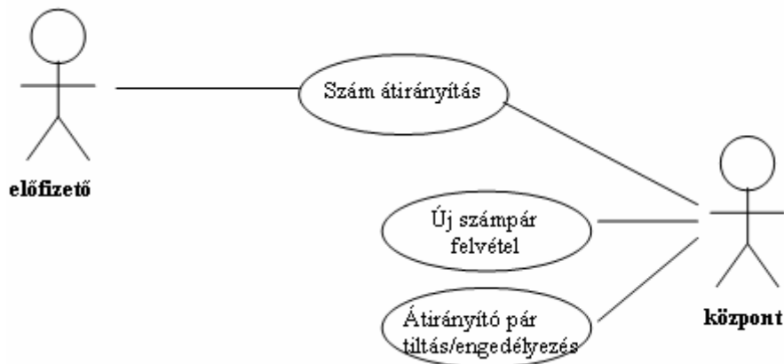
6.3. ábra: A telefonközpont használati eset diagramja.
