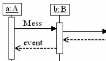
7.1. ábra: Üzenetek implementációja metódusként.
