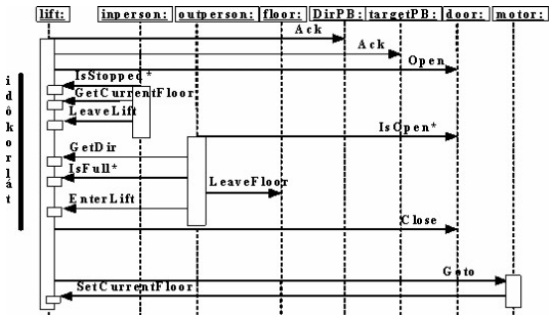
8.11. ábra: A működés a lift szemszögéből.
