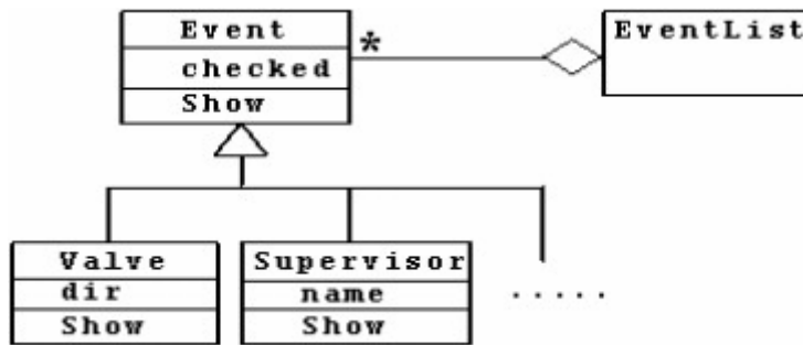
6.29. ábra: A folyamat-felügyelő rendszer osztálydiagramja.
