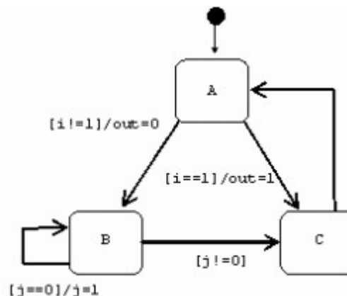
7.2. ábra: Példa állapotgép.
