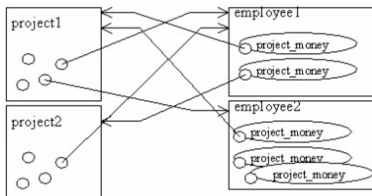
7.10. ábra: m-n asszociáció.
