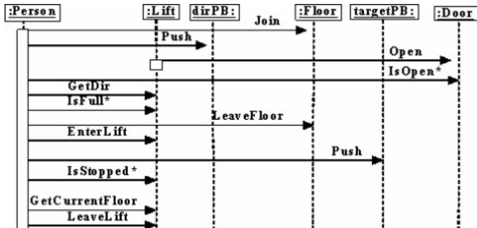
8.10. ábra: A működés az utazók szemszögéből.
