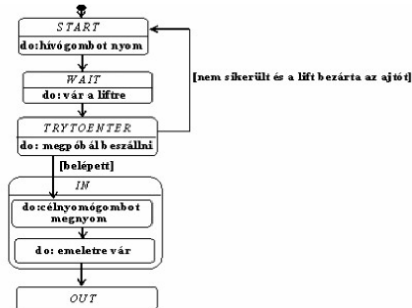
8.14. ábra: A személy állapottér modellje.
