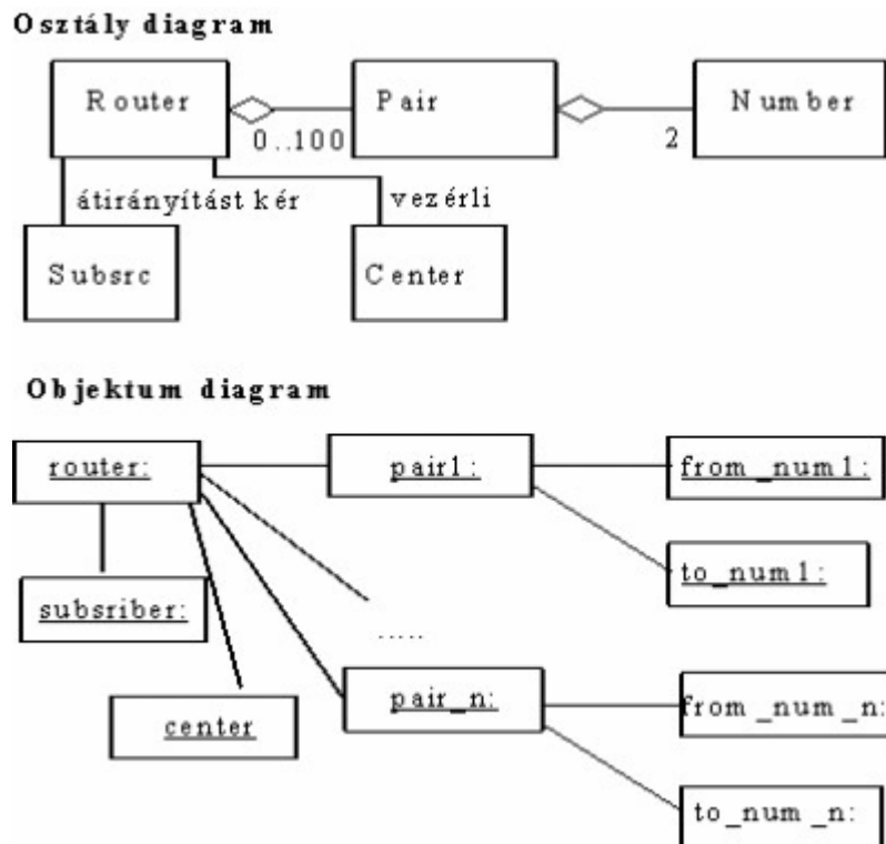
6.4. ábra: A hívásátírányító rendszer osztály és objektum modellje.
