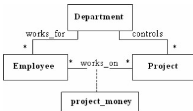
7.6. ábra: A tanszék objektum-modellje.
