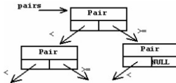
6.28. ábra: A párok bináris fában.
