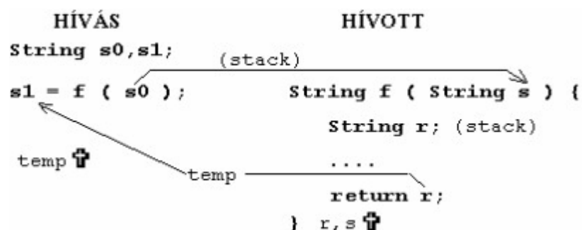
6.2. ábra: Paraméter és eredmény átadása a hívó és hívott függvény között.
