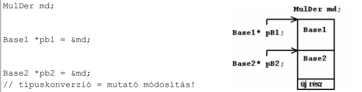
6.26. ábra: Szűkítő típuskonverzió többszörös öröklés esetén.
