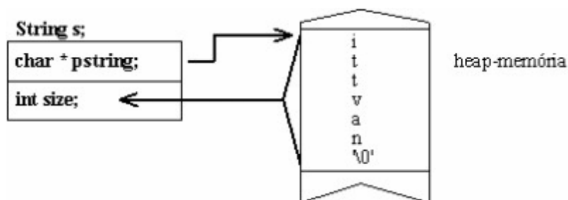
6.1. ábra: A sztring memóriaképe.
