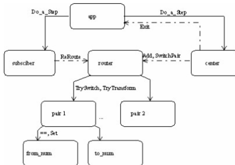
6.16. ábra: Az objektumok kommunikációs diagramja.
