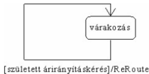
6.12. ábra: A router objektum dinamikus modellje átirányítás kérés esetén.
