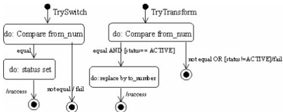
6.8. ábra: A pár objektum dinamikus modellje
