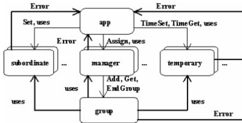
8.7. ábra: Az objektumok láthatósági igényei.
