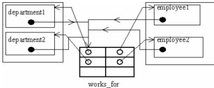
7.9. ábra: Asszociációs objektum.
