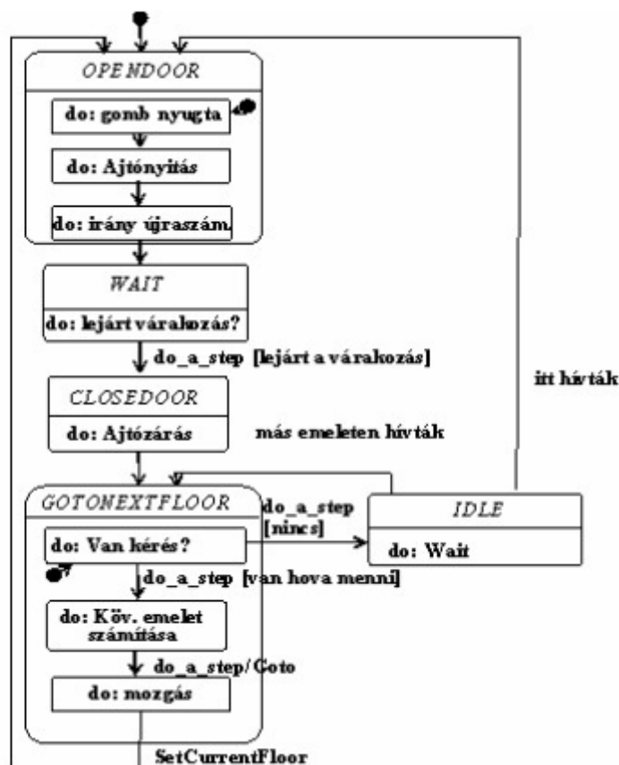
8.16. ábra: A Lift módosított állapotgépe
