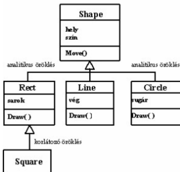
6.18. ábra: Geometriai alakzatok öröklési fája.
