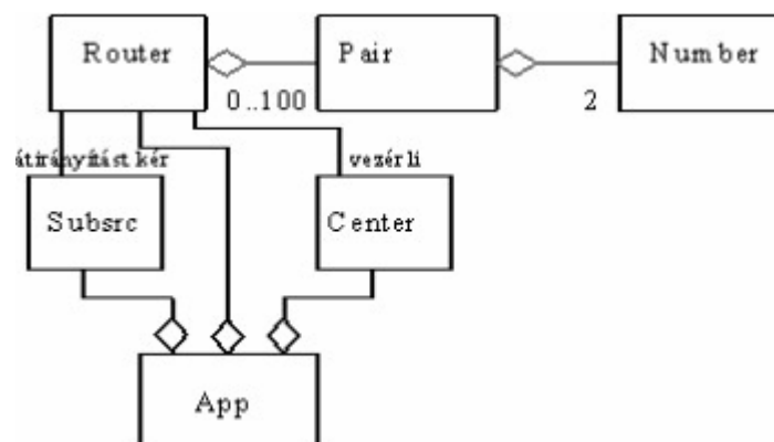
6.14. ábra: A tervezési szempontokat figyelembe vevő osztálydiagram.
