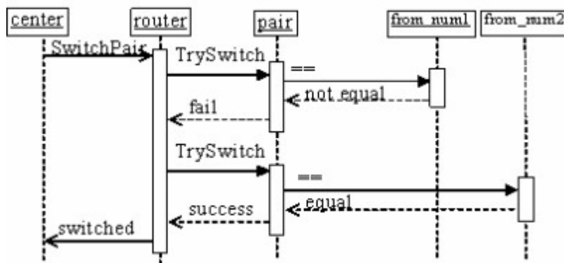
6.6. ábra: Szám tiltása/engedélyezése
