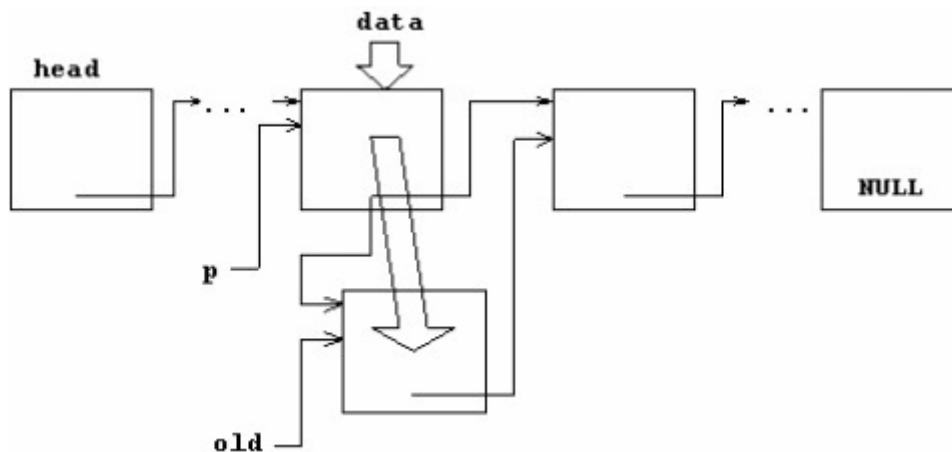
6.31. ábra: Beszúrás egy stázsát használó láncolt listába.
