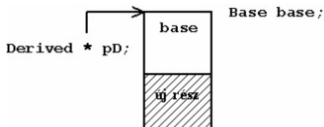
6.25. ábra: Bővítő típuskonverzió.
