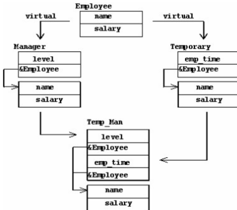
6.23. ábra: A többszörös öröklés adattag többszörözésének elkerülése virtuális bázis-osztályok alkalmazásával.
