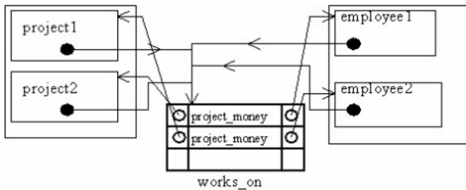
7.11. ábra: m-n asszociáció asszociációs objektummal.
