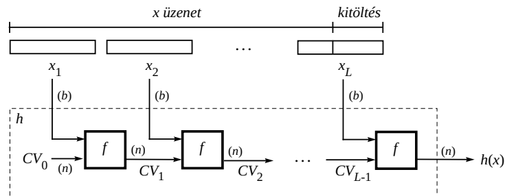
3.15. ábra. Az iteratív hash függvény működésének vázlata.
