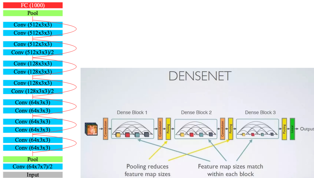
9.14. ábra. A ResNet (bal) és a DenseNet (jobb) modellek.
