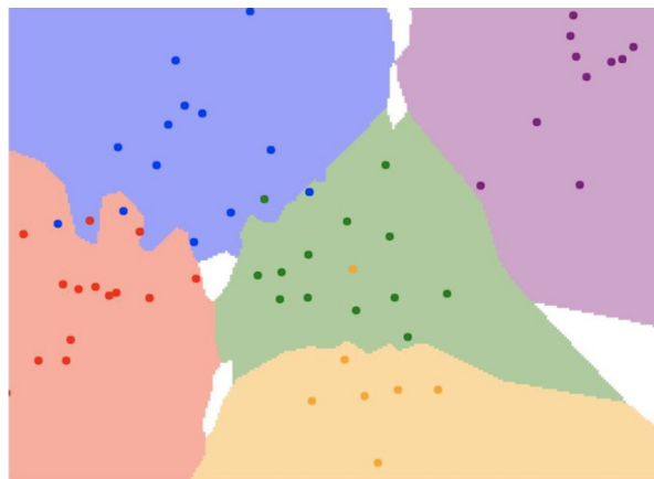
8.2. ábra. A k NN algoritmus döntési területei k = 3 esetében.
