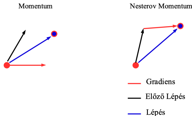
8.7. ábra. A momentum módszer (bal) és a Nesterov-momentum (jobb). Ez utóbbi előbb lép a momentum irányba, majd ott számolja ki a gradienst, ami valamivel stabilabb működést eredményez.
