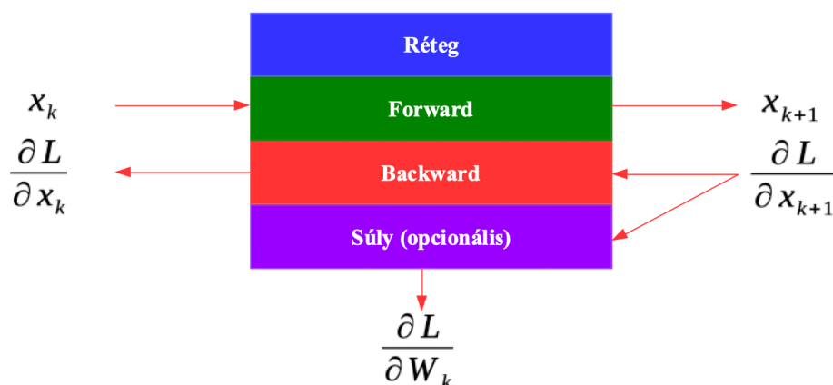
8.11. ábra. Egy réteg által biztosított, általános interfész, ami tartalmazza a tanításhoz és a predikcióhoz szükséges komponenseket is.
