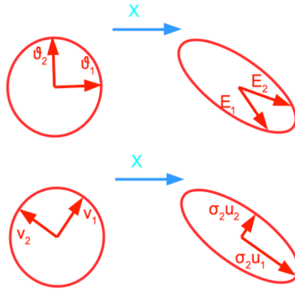
13.7. ábra. A szinguláris vektorok és értékek: A TLS algoritmus során az egységkör vektorai közül keressük azt, amelyik hossza a mátrixszorzás után a lehető legkisebb lesz. Ha veszünk az egységkörtől egy ortogonális vektorrendszert, akkor ezek segítségével lineáris kombinációkkal előállítható az összes transzformált vektort tartalmazó ellipszoid (felül). Ha létezne egy olyan vektorrendszer, amely a mátrixtranszformáció előtt és után is ortogonális lenne, könnyen belátható, hogy ezek pont a kapott ellipszoid főtengelyeivel esnének egybe. Ezt a vektorrendszert hívjuk szinguláris vektoroknak, mely a sajátvektorok általánosításának tekinthetők.
