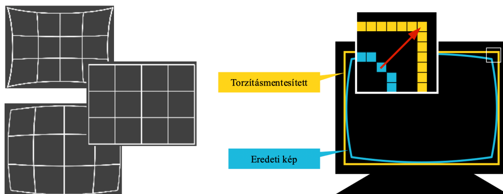
13.9. ábra. A lencsetorzítást gyakran egy lookup table segítségével korrigáljuk. Meghatározás után minden pixel esetére meghatározzuk azt, hogy a torzításmentesítés után hova kellene kerülnie, majd e térkép segítségével már gyorsan elvégezhetjük a képek torzításmentesítését.
