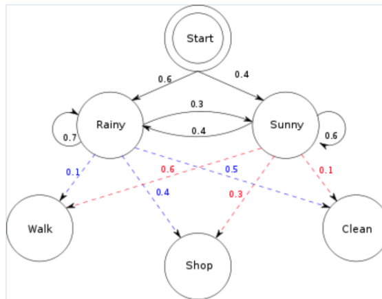
5.14. ábra. A Rejtett Markov-Modell: ebben a példában a rejtett állapotok az időjárást írják le, a megfigyelések pedig egy adott ember napi tevékenységeit.
