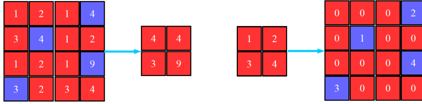
11.4. ábra. A max pooling művelet.
