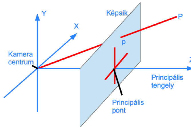
13.3. ábra. A pinhole kamera geometriai modellje. Érdemes megjegyezni, hogy ezen a modellen a képsík már a pinhole előtt található: így módon álló képet kapunk. Ez természetesen csak matematikai egyszerűsítés.
