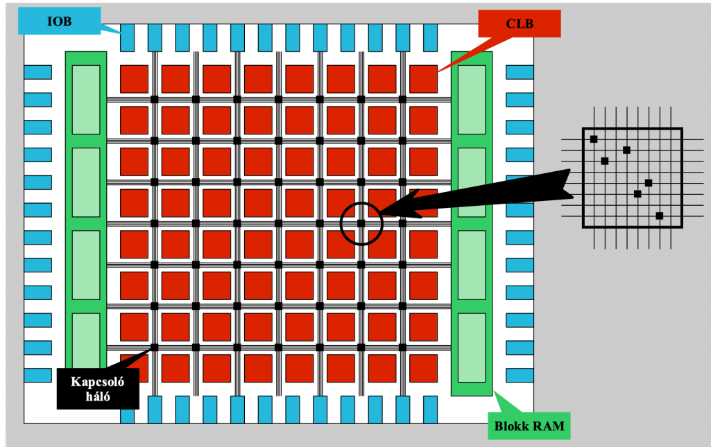
17.8. ábra. Az FPGA általános felépítése.
