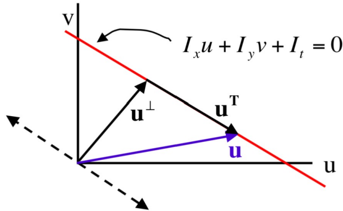
5.10. ábra. Az intenzitás-áramlás egyenlet által meghatározott megoldáshalmaz (piros egyenes), a megoldás komponensei.
