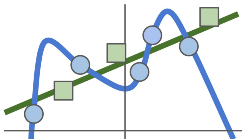
8.1. ábra. Az overfitting egy dimenzió esetén. Látható, hogy a kék színű modell rátanul a tanító adatbázisban lévő zajra, így a tesztadatokon (zöld) rosszul teljesít.
