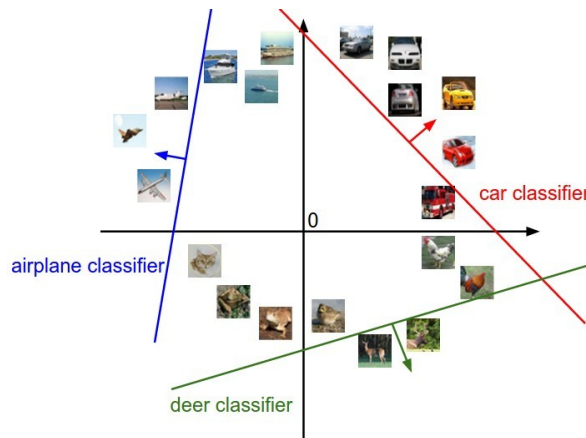
8.5. ábra. A lineáris osztályozás esetében az egyes osztály jósági értékek a tér egy irányában lineárisan nőnek, míg a többiben konstansak. A növekedés irányát a súlymátrix adott osztályhoz tartozó sorvektora határozza meg.
