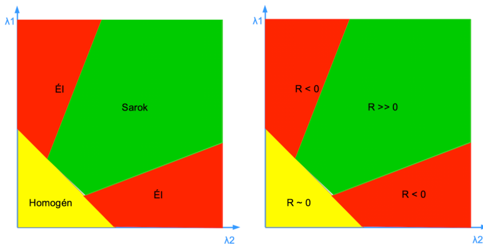
4.4. ábra. A KLT (bal) és a Harris (jobb) sarokság értékek osztályozási elve.
