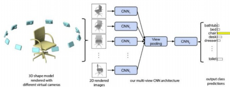
15.14. ábra. A Projekció alapú mély tanulás sémája.
