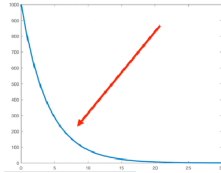
6.7. ábra. A klaszterek számának megválasztása. Bár a klaszterezés hibája monoton csökken, érdemes az ábrán jelölt könyökpontot választani, hiszen eddig érünk el jelentős javulást a klaszterszám növelésével.
