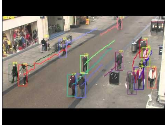
5.6. ábra. Objektumkövetés.
