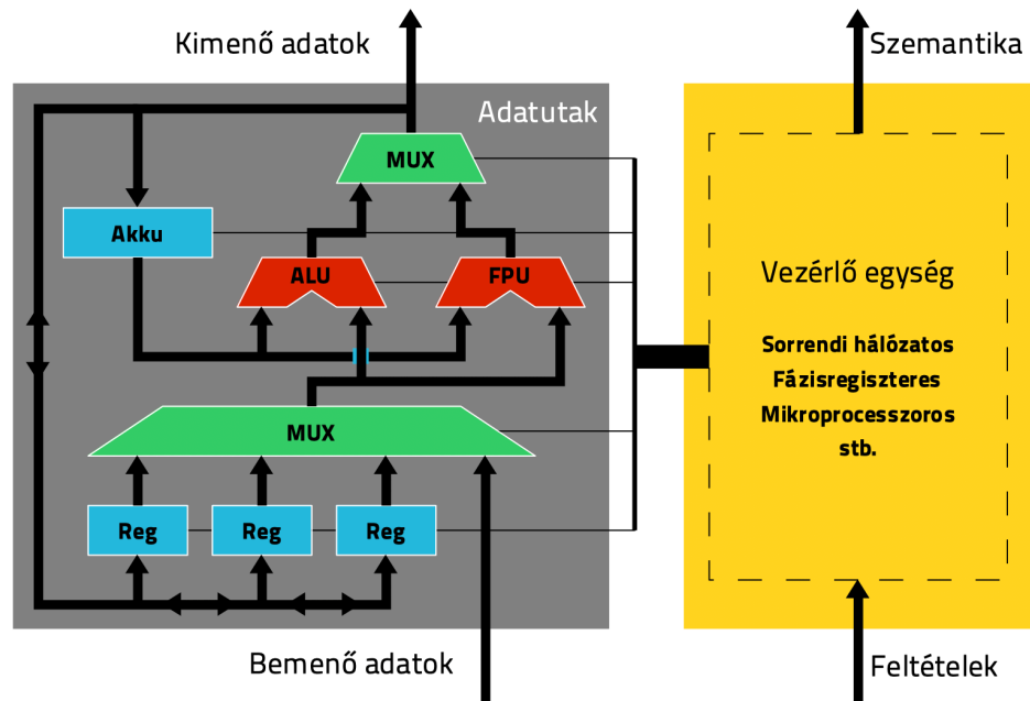
17.15. ábra. Az adatutak rendszere.
