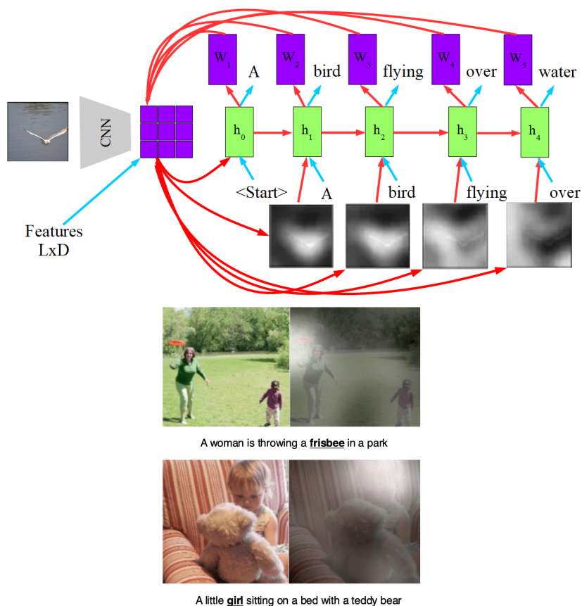
12.7. ábra. A puha figyelem elve (bal) és hatása a feliratozásra (jobb). Ezeken a képeken a háló által generált figyelem súlyok látszanak az aláhúzott szó kiadásának időpillanatában
