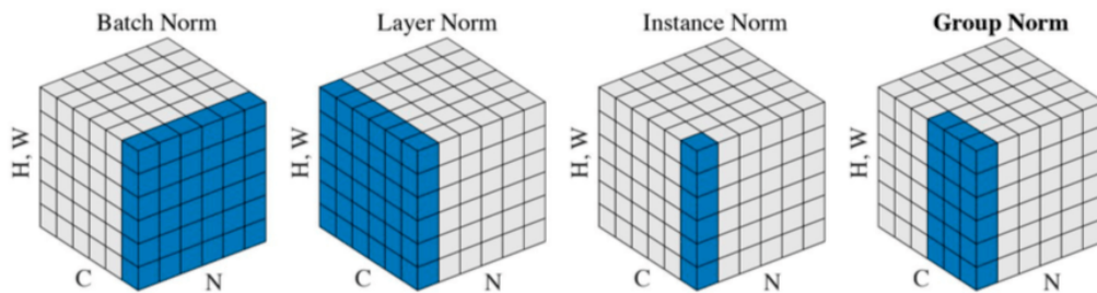
10.7. ábra. Érdeemes megjegyezni, hogy a batch normalizáción kívül létezik még réteg (layer) normalizáció, ahol a teljes aktivációs tömböt normalizáljuk egyedenként külön. Egyed (instance) normalizáció esetén az egyes csatornákat külön-külön normalizáljuk a térbeli dimenziók mentén. A kettő közti kompromisszum a csoport normalizálás, ahol néhány csatornát egybe veszünk.
