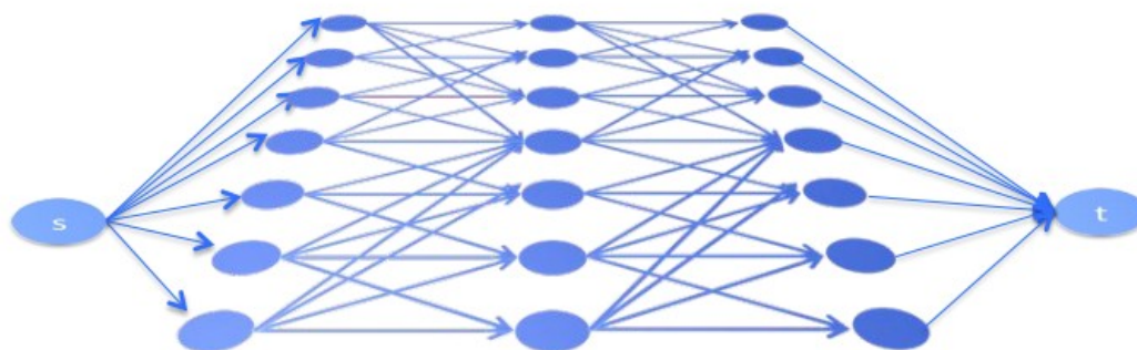
5.17. ábra. A több képkockán történő követés gráfja. A gráf minden szintje egy képkockához tartozik, minden szinten egy csomópont pedig egy objektum észlelés.
