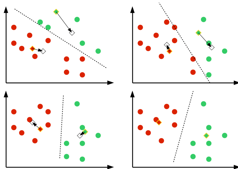
6.6. ábra. A k-means elve.
