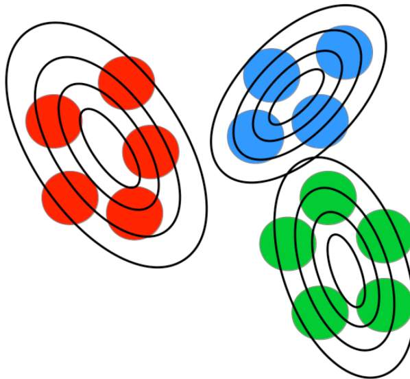
6.8. ábra. A MoG klaszterezés elve. Az ábrán az egyes klasztereket leíró gauss eloszlások szint-vonalait láthatjuk.
