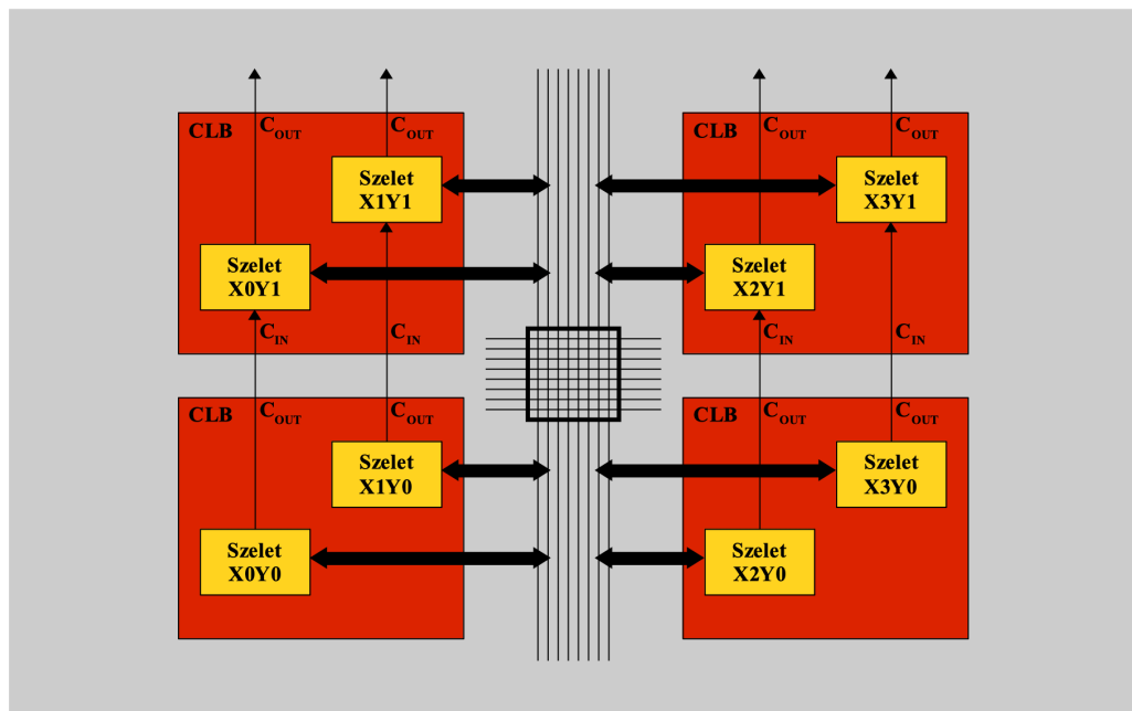
17.9. ábra. A CLB-k általános felépítése.
