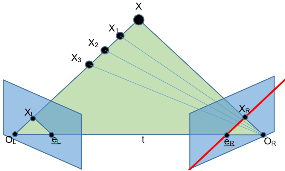
13.10. ábra. Az epipoláris elrendezés.
