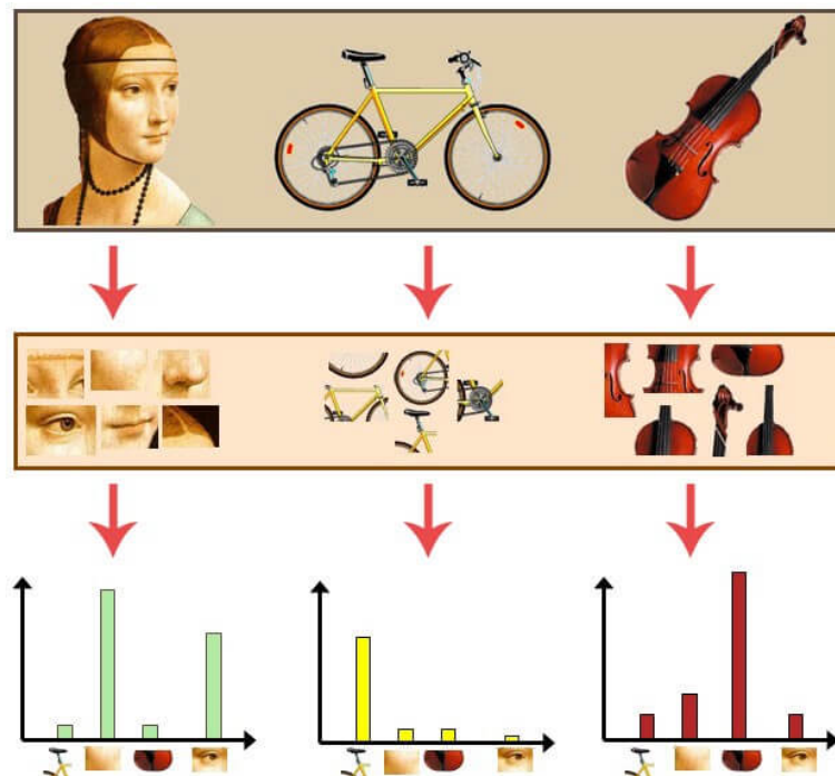
5.3. ábra. A vizuális szavak modellje.
