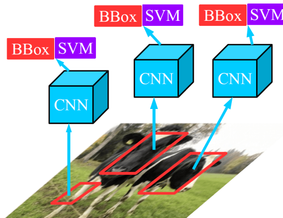
11.8. ábra. A R-CNN architektúra.
