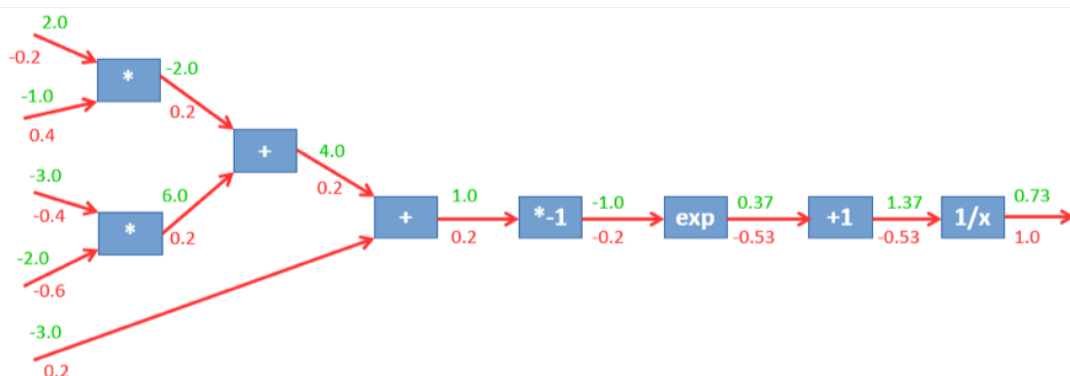
8.10. ábra. A backpropagation végrehajtása egy példa gráfon. Zölddel az aktivációk, pirossal a deriváltak szerepelnek.
