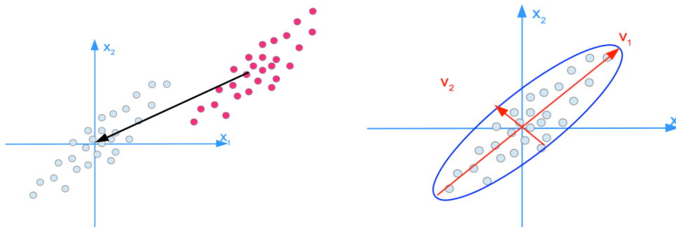
4.12. ábra. A redukálendő adathalmaz normálása (bal), és a kapott főkomponensek (jobb).
