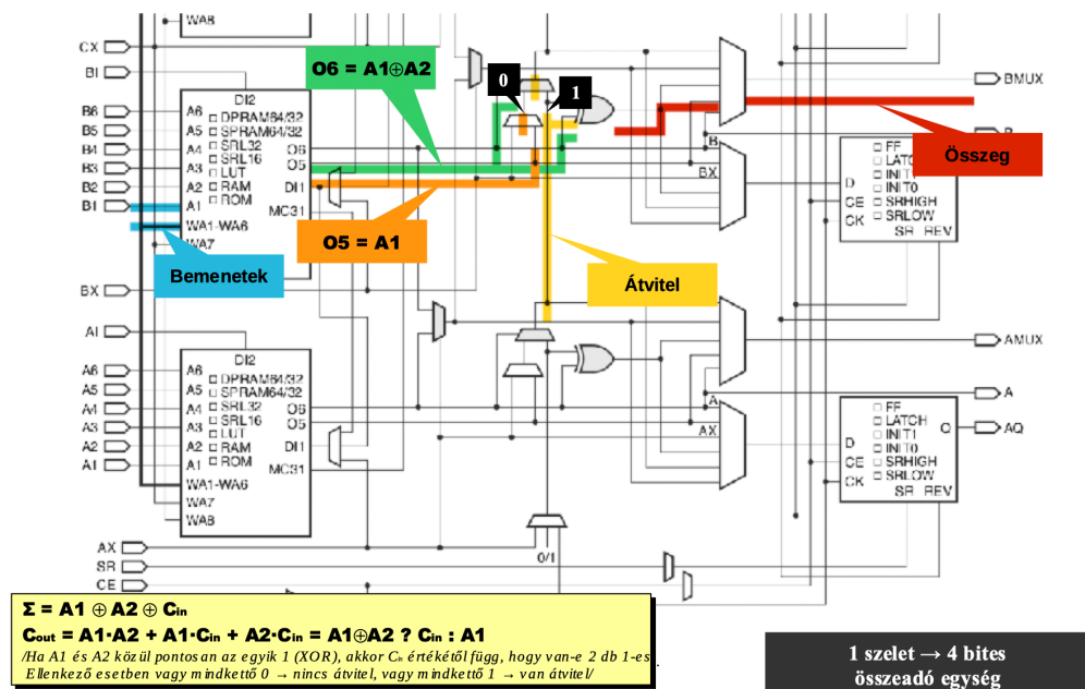
17.11. ábra. Az összeadás megvalósítása.
