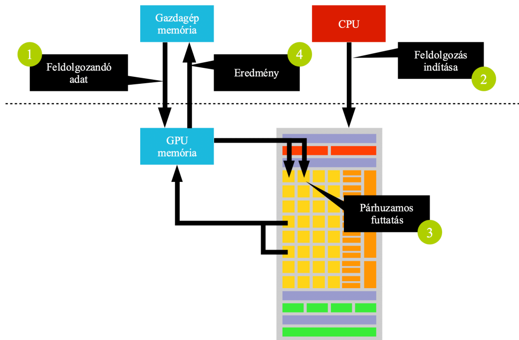
16.6. ábra. A GPU program futásának módja.
