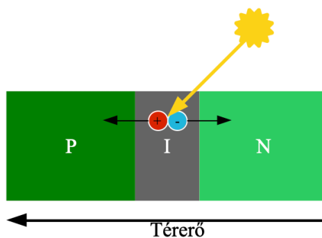
1.5. ábra. A fotodióda működési elve.
