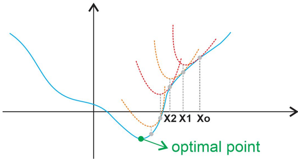
8.8. ábra. A Newton algoritmus elve.
