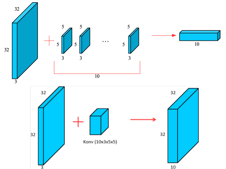
9.1. ábra. A konvolúció végreajtása egy kép tömbön több szűrővel (felül), és az ezzel ekvivalens konvolúciós réteg (alul).
