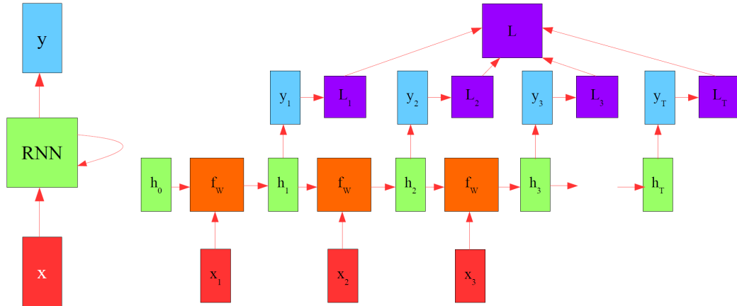
12.2. ábra. Egy RNN cella felépítése (bal) és időbeli kibontása (jobb).
