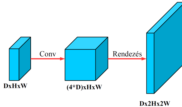
11.6. ábra. A sűrű felskálázó konvolúció (DUC).
