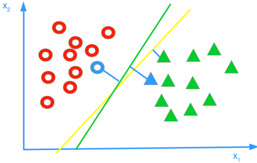
8.4. ábra. A bináris osztályozási feladat: A két osztály, az elválasztó hipersík, a support vektorok és a margin.
