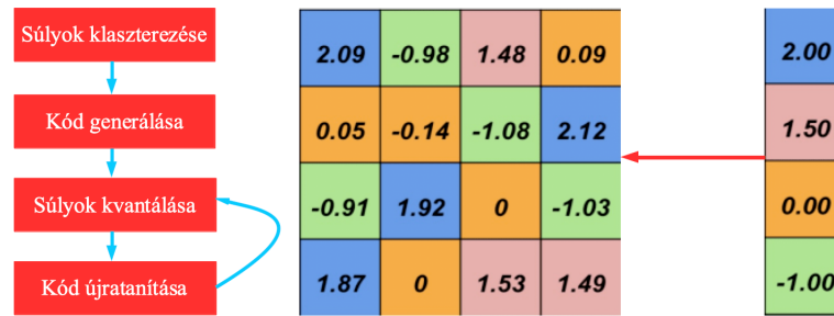
10.12. ábra. A Weight sharing módszere (bal) és a súlyok kvantálásának sémája (jobb).
