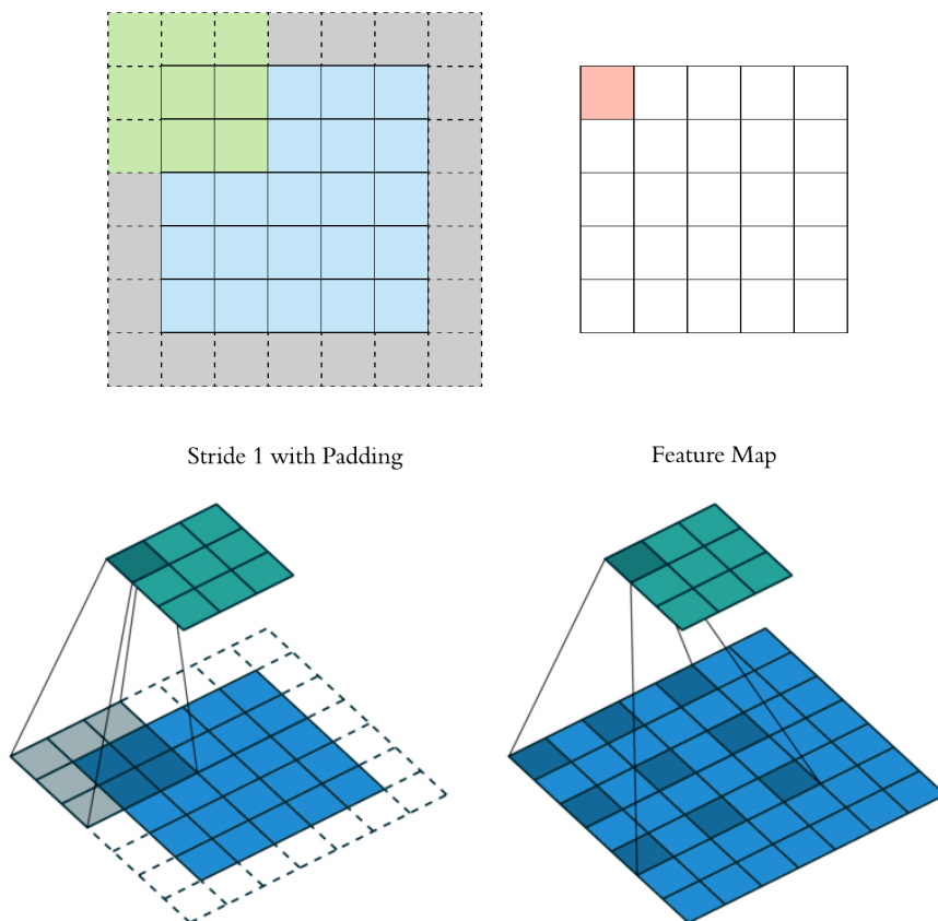
9.2. ábra. A padding (felül), a stride (alul bal) és a dilatació (alul jobb) hatása a konvolúció műveletére.
