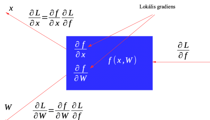
8.9. ábra. A láncszabály szemléltetése.
