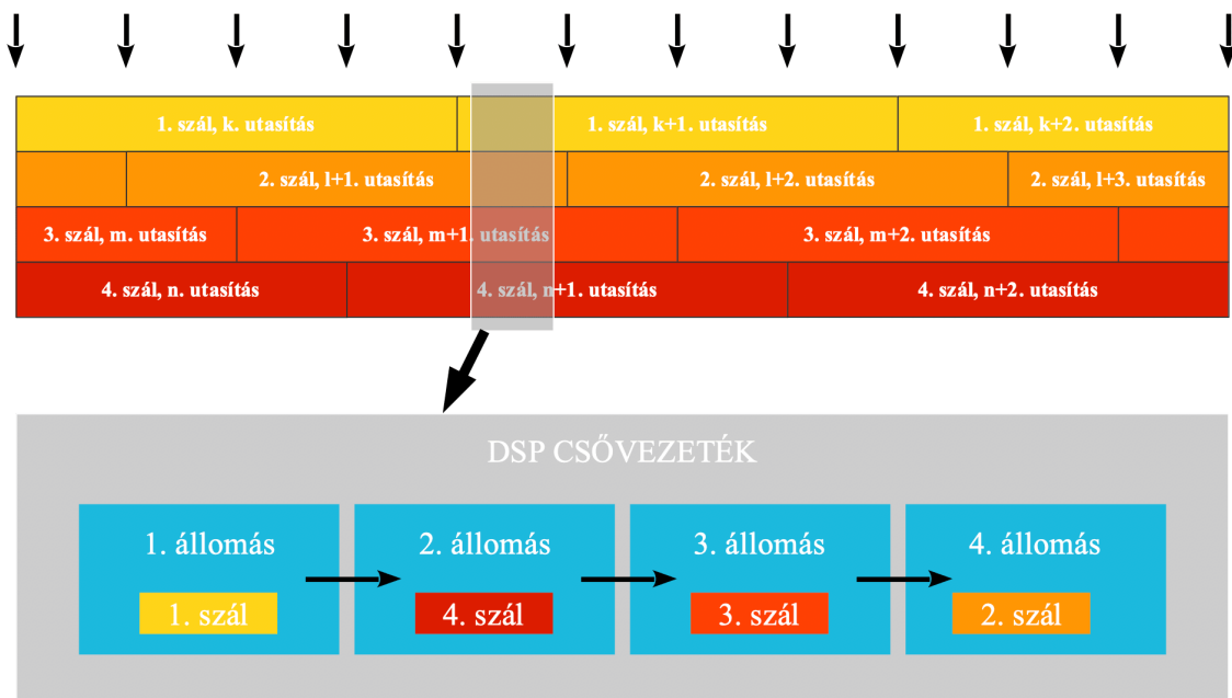
16.9. ábra. A csővezeték többszálú futásra való használata.
