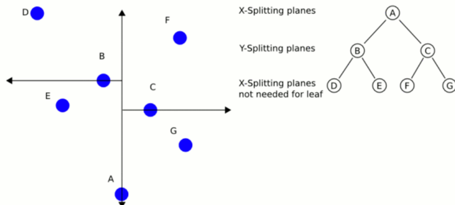
15.5. ábra. A kd-fa konstruálási szabálya.
