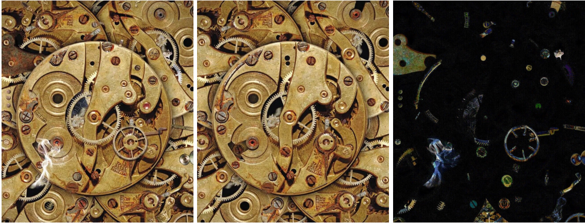
2.19. ábra. Különbségképzés.
