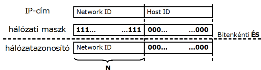
4. ábra. Hálózati cím előállítása hálózati maszk segítségével
